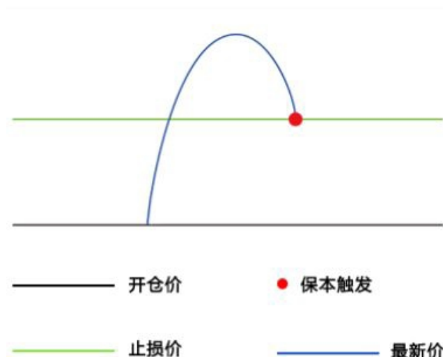
图 3.5.6.2 做多保本止盈原理
