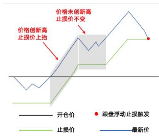
图 3.5.6.1 做多浮动止损原理
